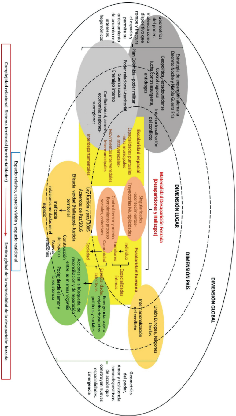
Figura 4. Complejidad relacional en el sistema territorial-territorialidades que define al sentido global de la desaparición forzada
